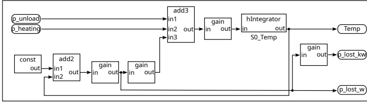
Abbildung 18: Teilmodell furnace
