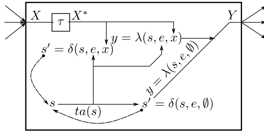
Abbildung 9: Dynamik eines atomaren NSA-DEVS
