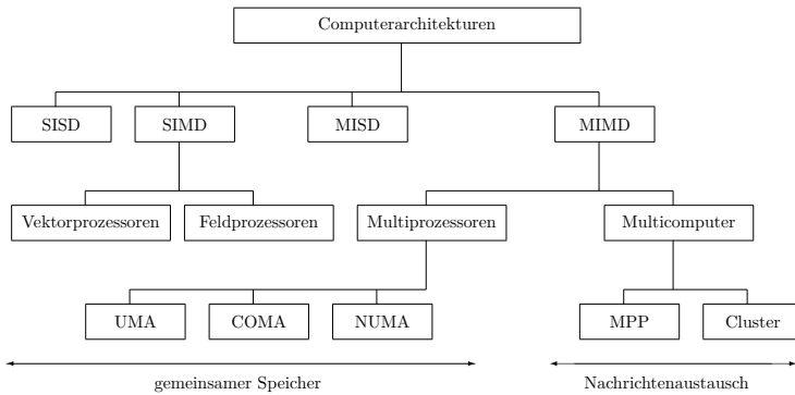
Abbildung 1: Computerarchitekturen nach [89].
