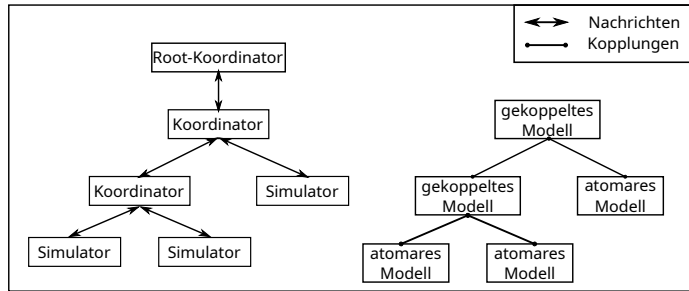
Abbildung 6: DEVS-Architektur
