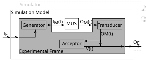
Abbildung 13: Aufbau des EF nach [107]
