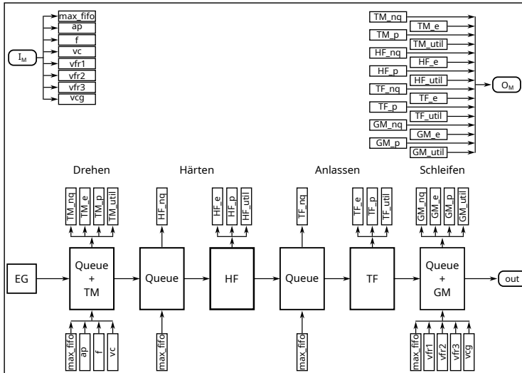
Abbildung 14: Struktur des MUS
