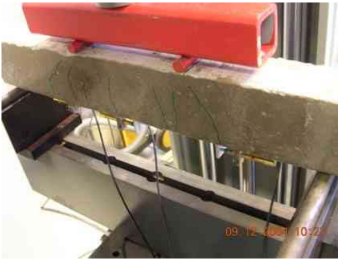
Belastung zwecks Risserzeugung
