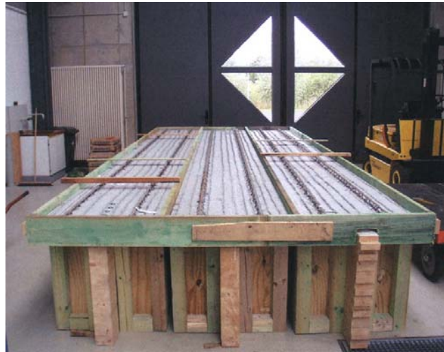
Betonage der 3 Prüfkörper
