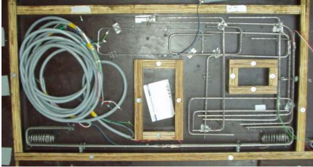
Bewehrungsführung 1. Wandscheibe
