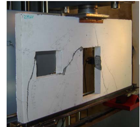
Rissverlauf 2. Wandscheibe
