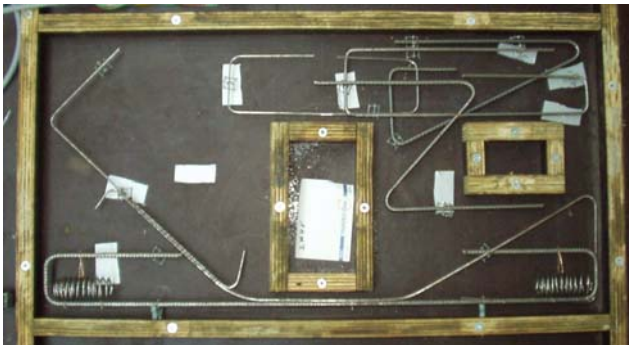
Bewehrungsführung 2. Wandscheibe
