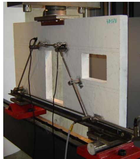
Prüfung 4. Wandscheibe
