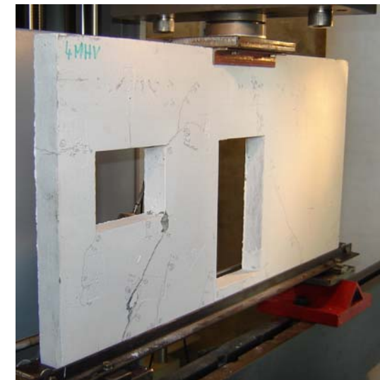
Rissverlauf 4. Wandscheibe
