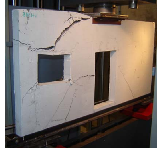
Rissverlauf 3. Wandscheibe
