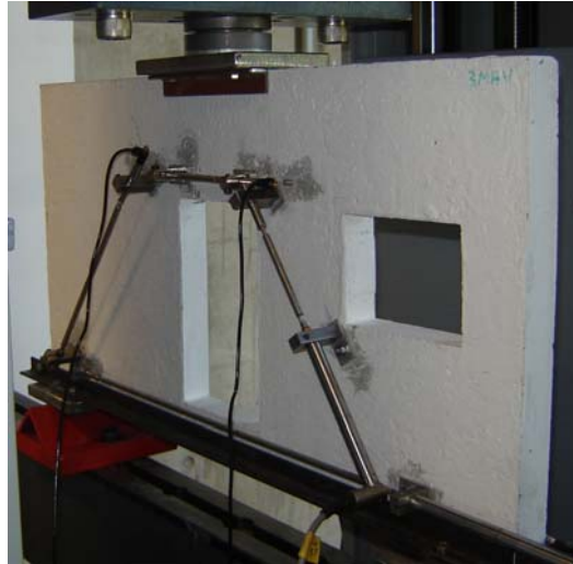
Prüfung 3. Wandscheibe
