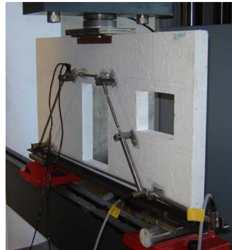
Prüfung 2. Wandscheibe
